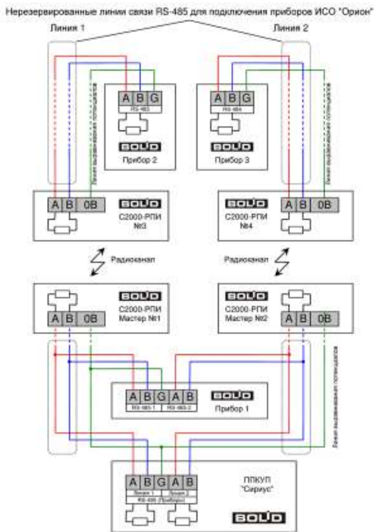
Рисунок 66. Схема подключения преобразователей нерезервированного интерфейса RS-485 «С2000-РПИ»
