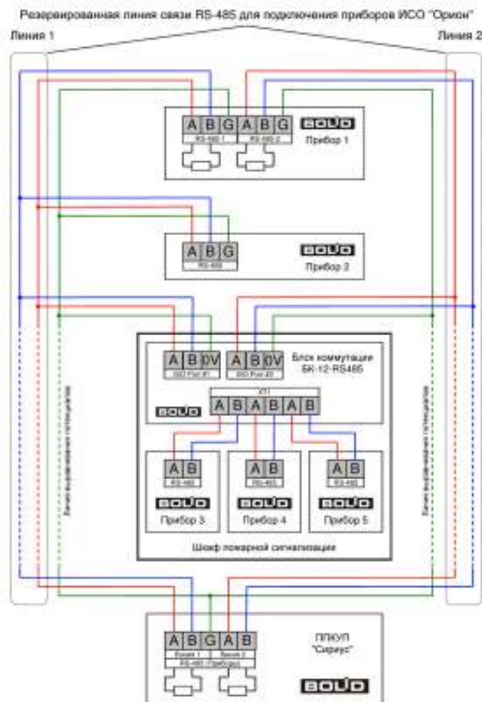
Рисунок 64. Схема подключения дополнительных блоков и приборов ИСО «Орион»
